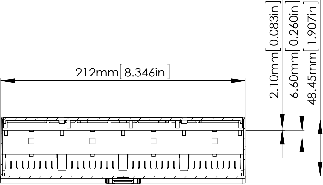
SECTION A-A
