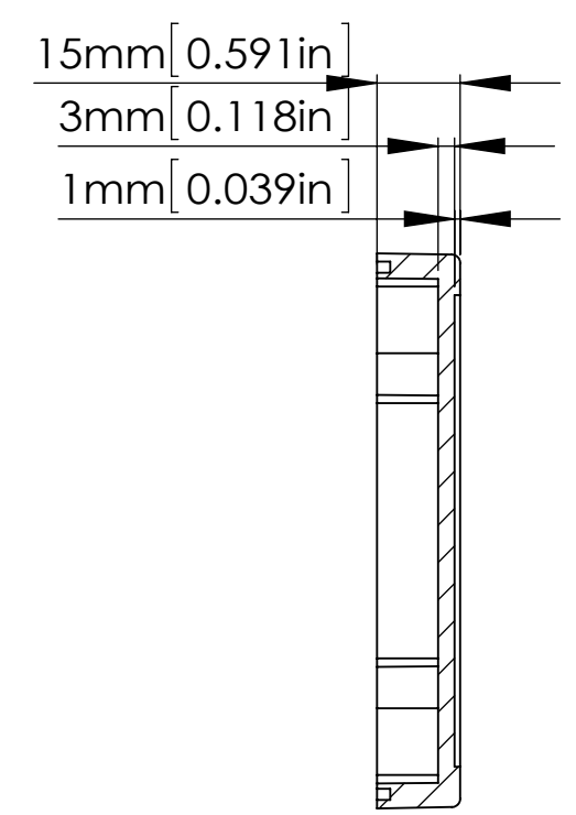
SECTION B-B SCALE 2 : 3
