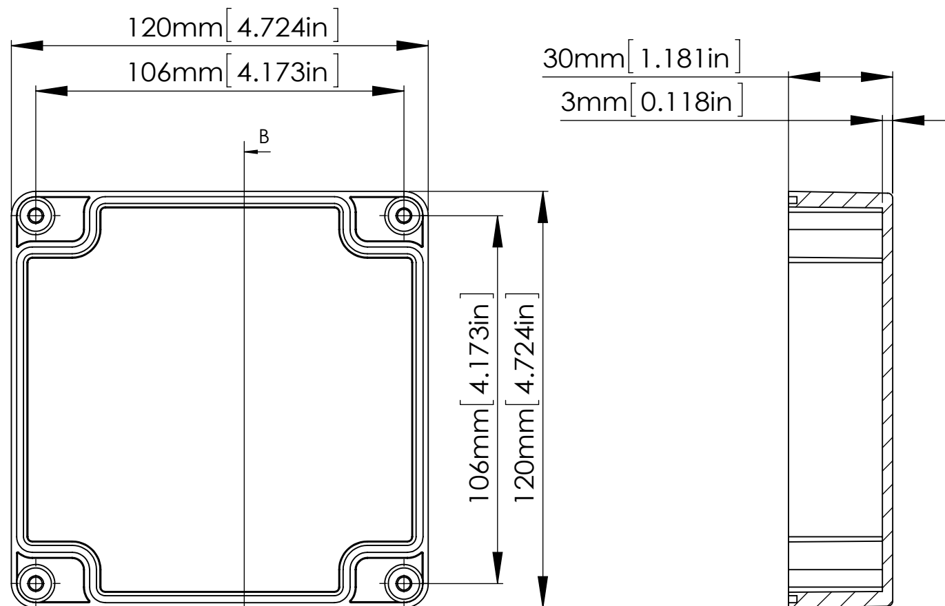
SECTION B-B SCALE 2 : 3
