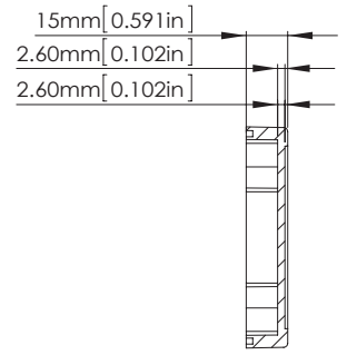
SECTION B-B SCALE 2 : 3
