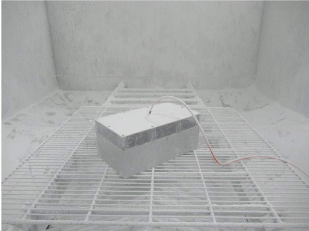
IP6X Test (G20583C-IP67)
