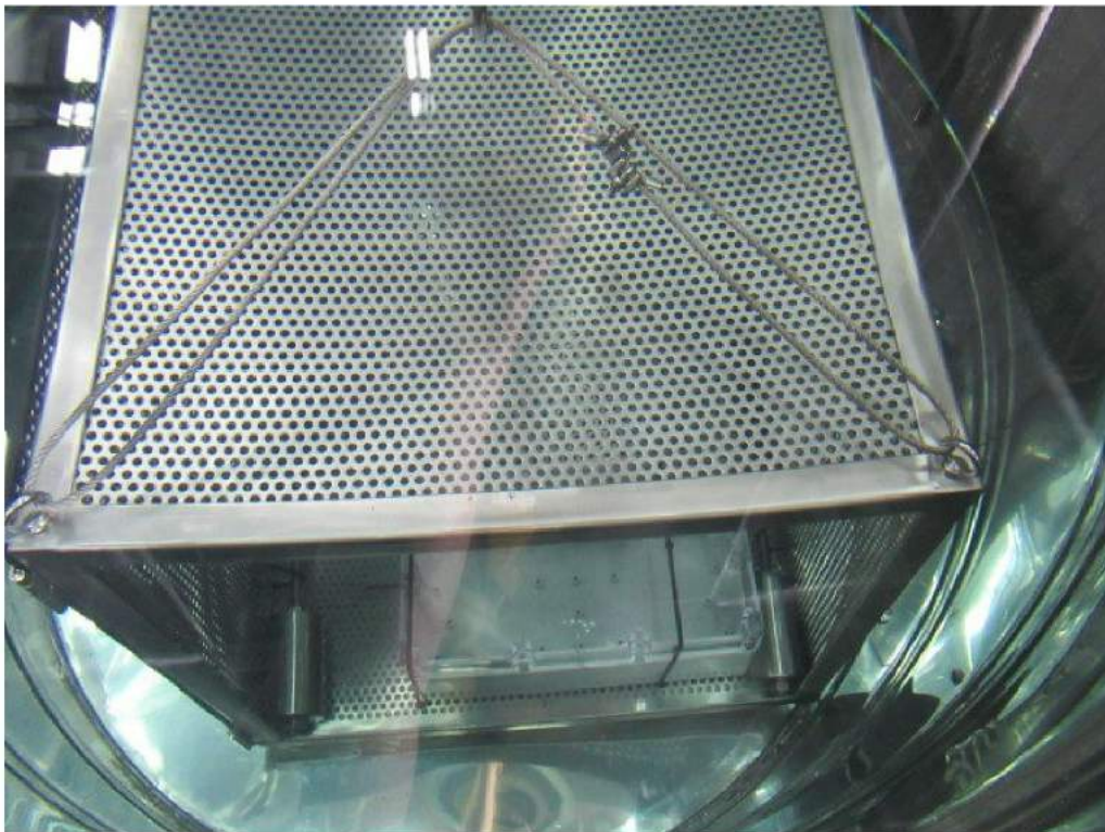
IPX8 Test (G20583C-IP67)
